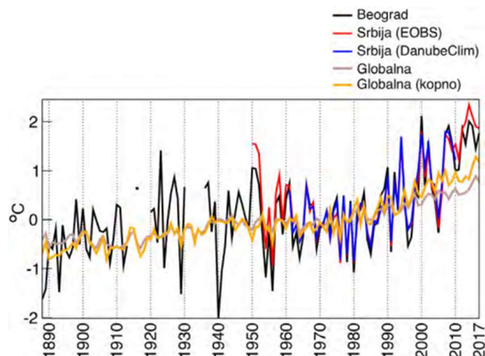
Слика 3.5. Одступање средње годишње температуре (°C) у односу на средњу вредност референтног периода (1961-1990.). Вредности за Београд добијене су из осматрања на метеоролошкој станици Опсерваторија Београд на којој постоји најдужи низ осматрања (од 1888. године). Просечне вредности за целу Србију добијене су из два сета података: E-OBS (база података са интерполираним дневним вредностима температура и падавина на резолуцији 10 km од 1950. године) и DanubeClim (база дневних интерполираних података резолуције 10 km за период 1961 - 2010. године)
