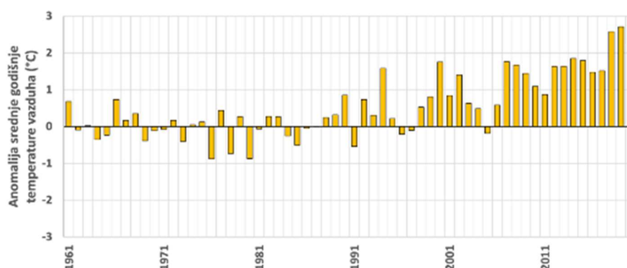
Слика 3.6. Одступања (аномалије) средњих годишњих температура ваздуха, осредњених за територију Републике Србије, за период 1961 – 2020. године у односу на средњу вредност референтног периода 1961 – 1990. године.
